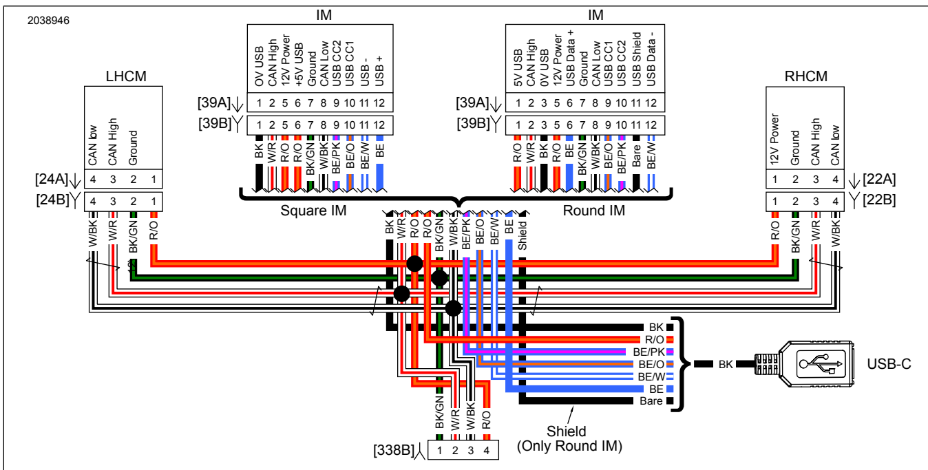
Figure 6. IM Circuit
