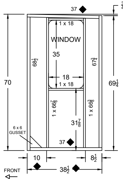
DINETTE ENDWALL (x2)
