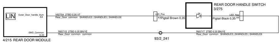
4/215 REAR DOOR MODULE
