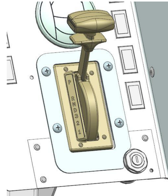
UTILIMASTER DASH
