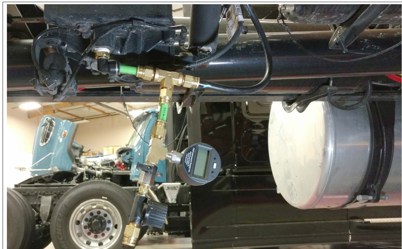
Fig. 4, Installation du manomètre à l'aide d'un pontage et d'un raccord en T
