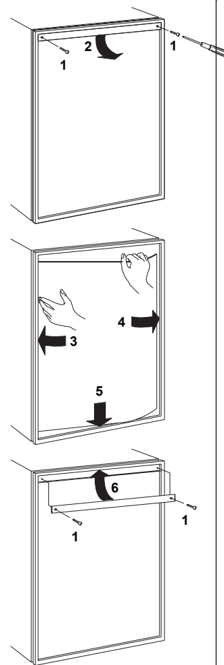
FIG 28 - DOOR PANEL
