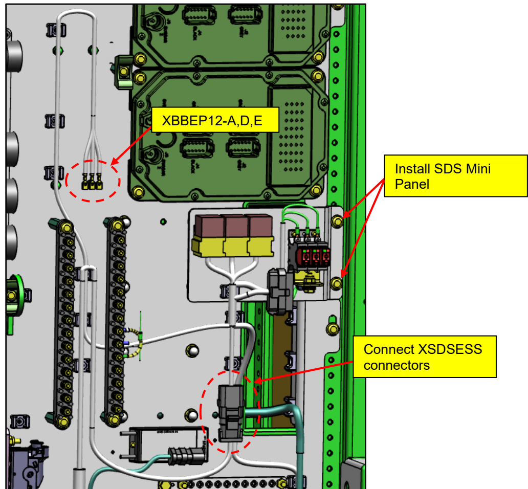
Figure 50: SDS Mini Panel
