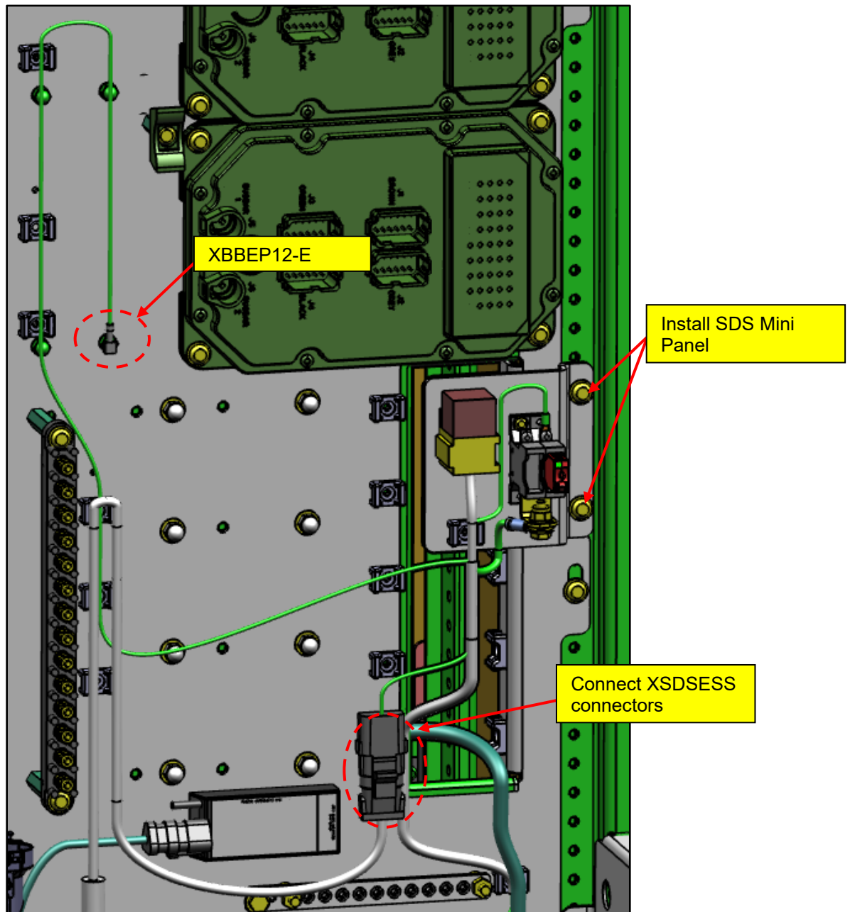
Figure 54: SDS Mini Panel
