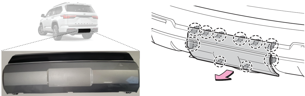
Cubierta del enganche para el remolque (Deseche después de retirarla)
