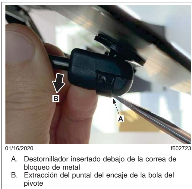
Fig. 1, Extracción del puntal del encaje de la bola
