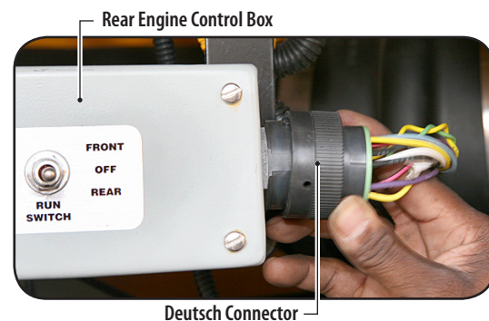
Deutsch Connector
