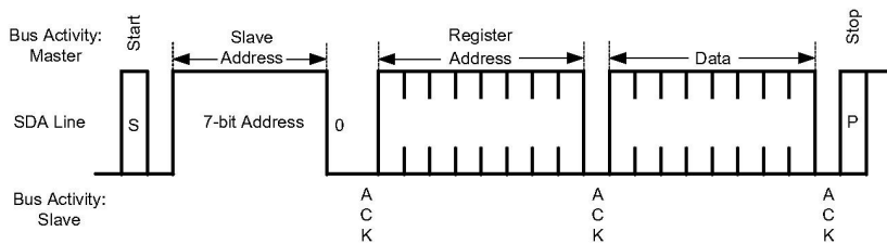
Figure 21. Write Byte
