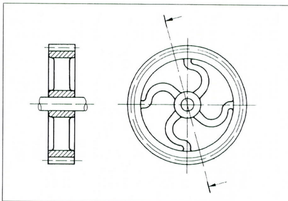
Fig. 8.21 Impact resistant web
