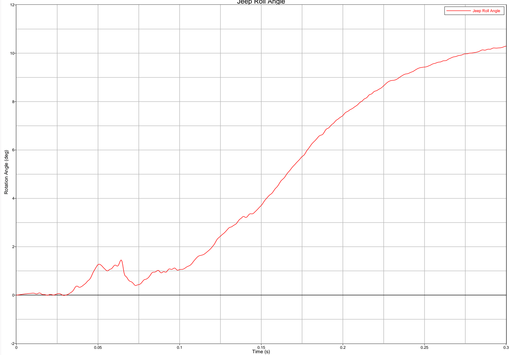
Jeep Roll Angle
