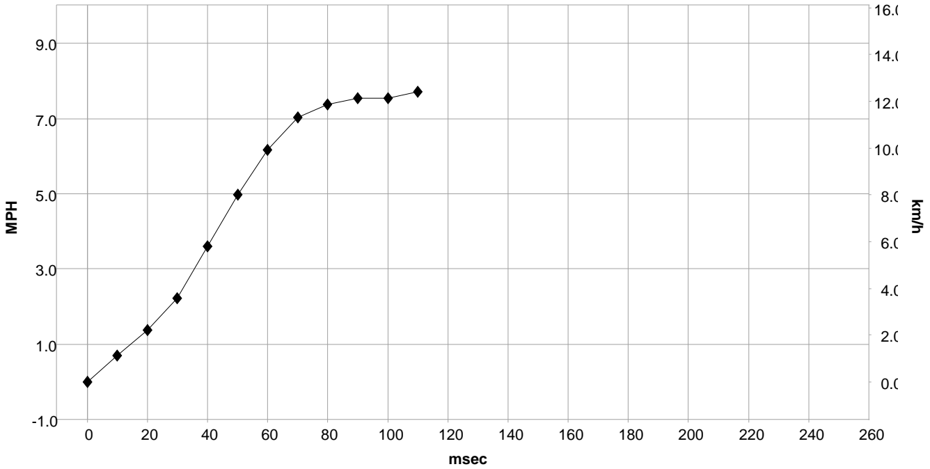
Longitudinal Delta-V
